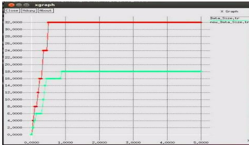
Fig. 5.4 Data size
